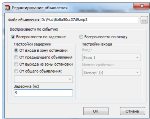
Рис.61. Добавление объявления для автоинформатора.
