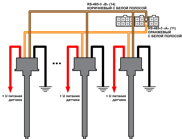
Рис.39. Схема подключения датчиков уровня топлива к дисплею.
