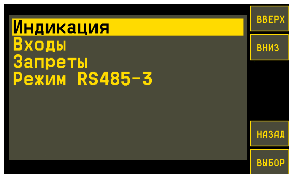
Рис.87. Меню «Управление».
