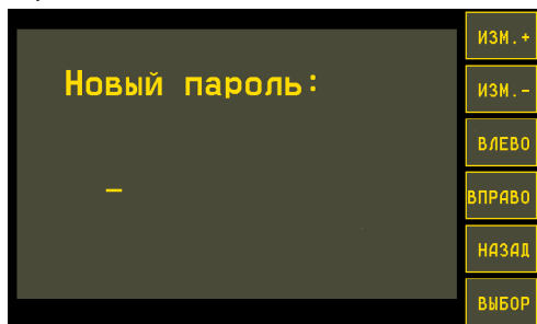
Рис.26. Изменение пароля.
