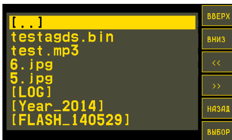
Рис.84. Содержимое SD-карты.
