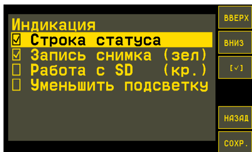
Рис.88. Управление индикацией.
