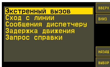
Рис.50. Темы сообщений.
