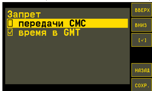
Рис.90. Установка запретов.
