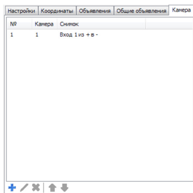
Рис.64. Вкладка «Камеры».
