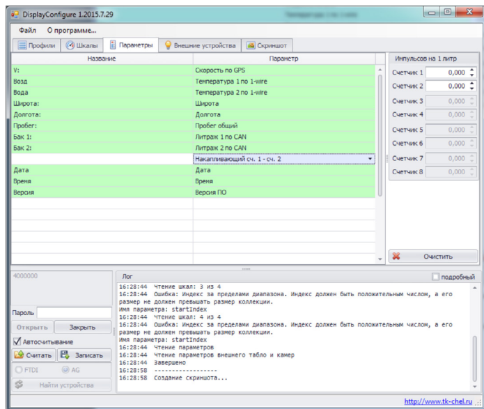
Рис.79. Вкладка «Параметры».
