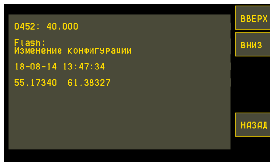
Рис.81. Журнал событий.
