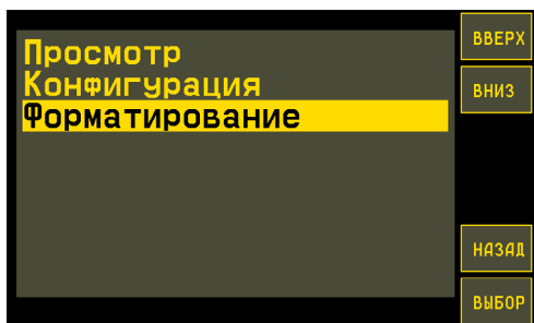
Рис.37. Форматирование SD-карты.
