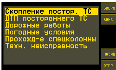
Рис.51. Сообщения.
