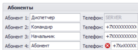
Рис.54. Список абонентов.
