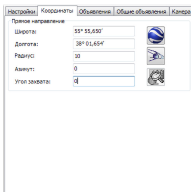
Рис.59. Вкладка «Координаты».
