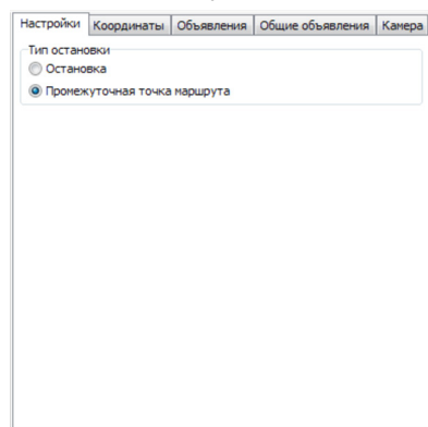
Рис.58. Вкладка «Настройки».
