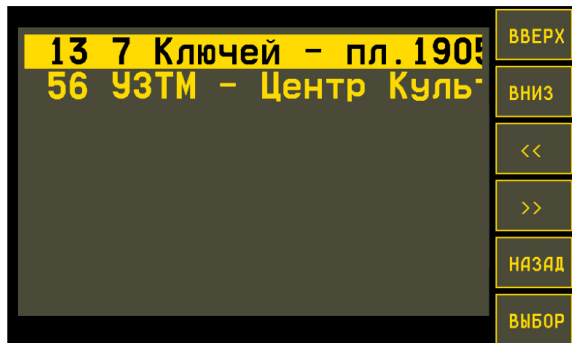
Рис.69. Выбор маршрута.
