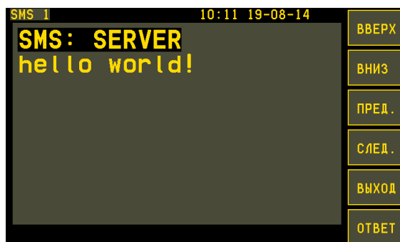
Рис.48. Входящее сообщение.
