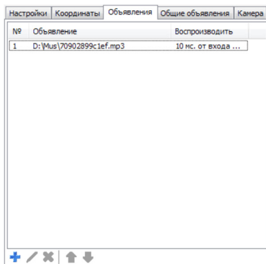
Рис.60. Вкладка «Объявления».
