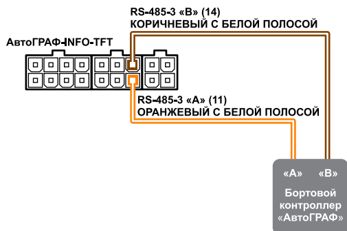
Рис.38. Схема подключения к контроллеру АвтоГРАФ.
