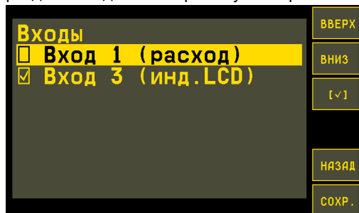
Рис.89. Управление входами.
