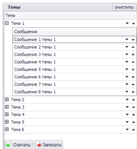
Рис.52. Формализованные сообщения.
