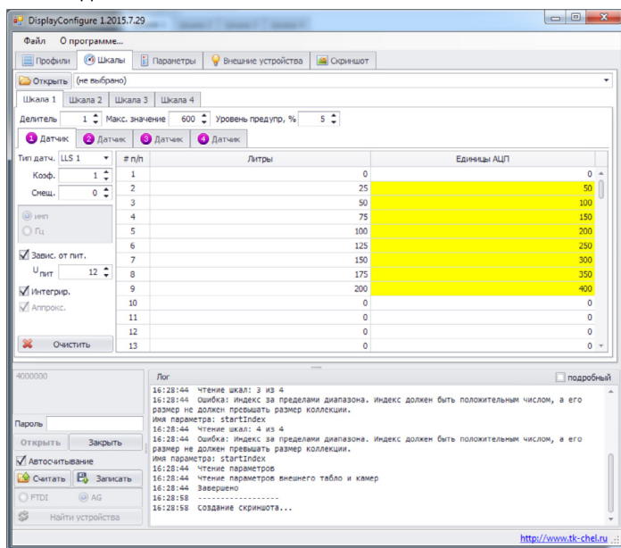
Рис.80. Вкладка «Шкалы».
