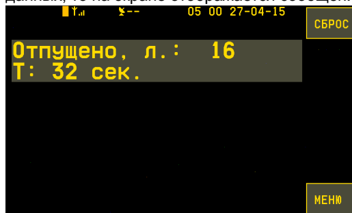
Рис.78. Показания топливозаправщика.
