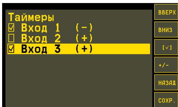
Рис.92. Настройка таймеров.
