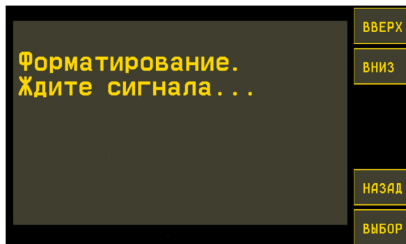
Рис.86. Форматирование SD-карты.
