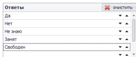
Рис.53. Быстрые ответы.
